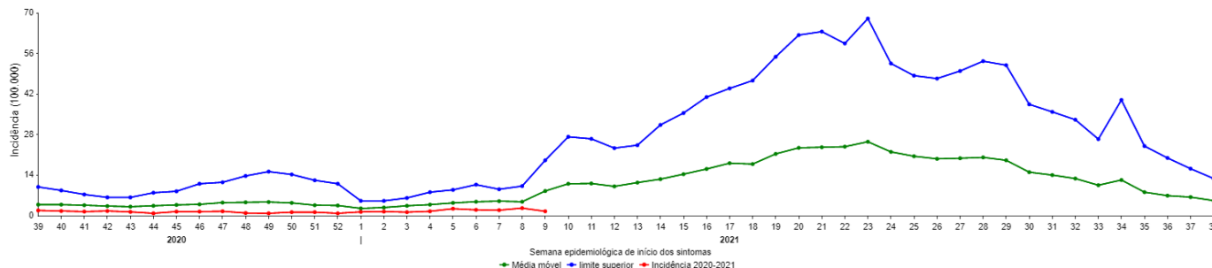
Figura 2 - Dengue: Diagrama de Controle, Fortaleza 2020 - 2021.
