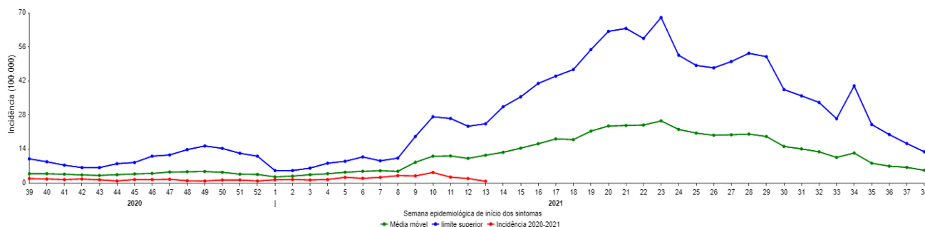
Figura 2 - Dengue: Diagrama de Controle, Fortaleza 2020 - 2021.
